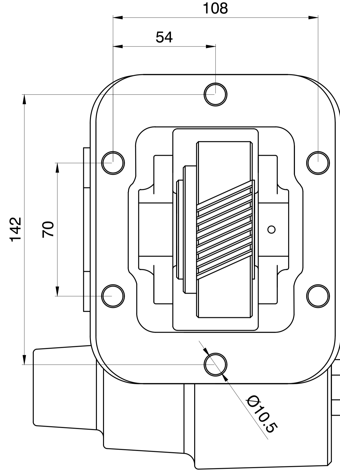
PTO Mil Dönüş Yönü Sağa (Saat Yönü)
