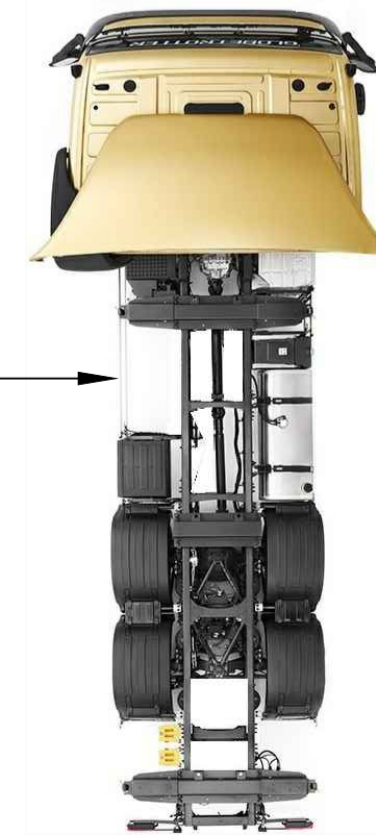
PTO Bağlantı Yeri Aracın Sol Yanı
