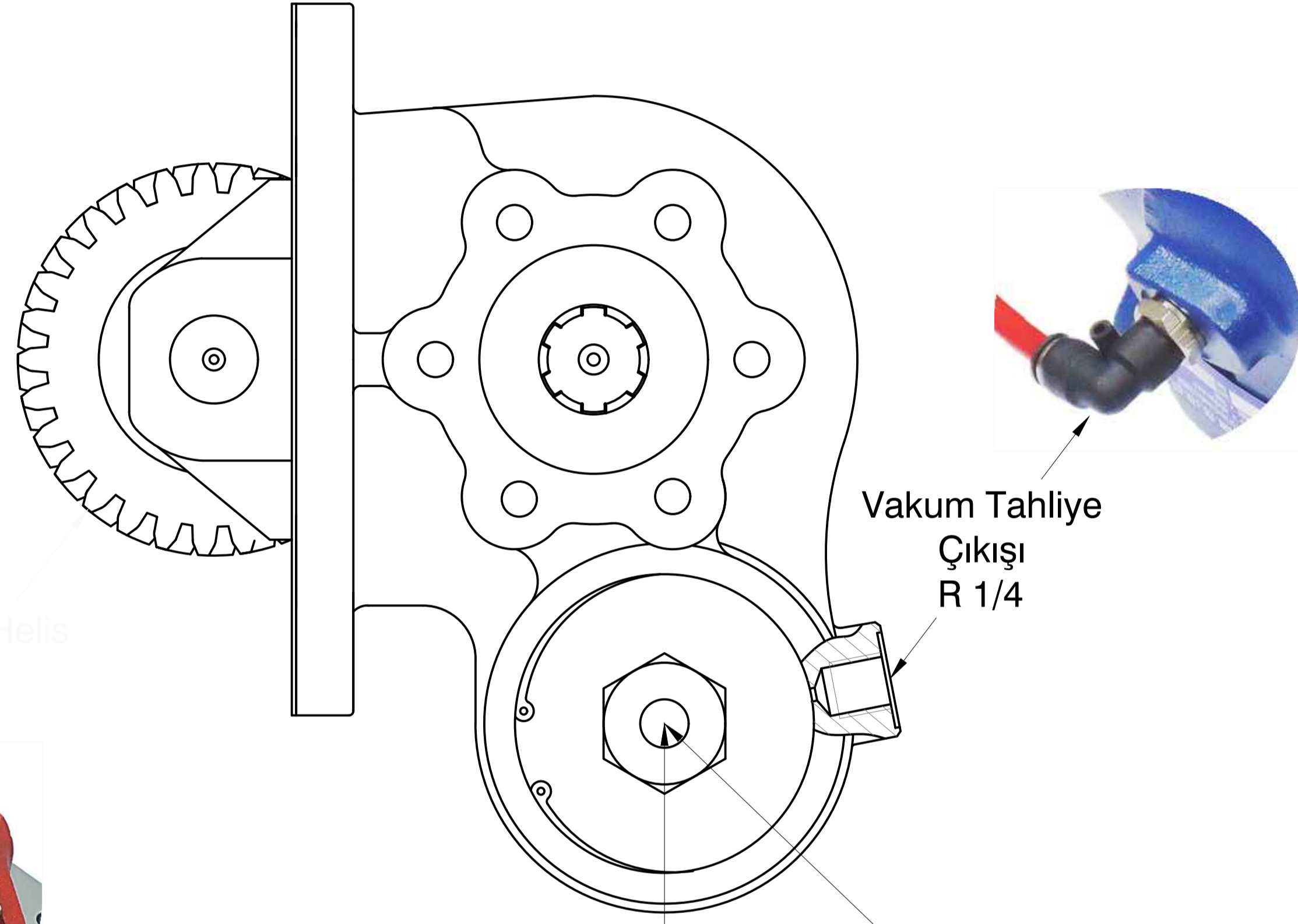
Vakum Girişi R 1/4
